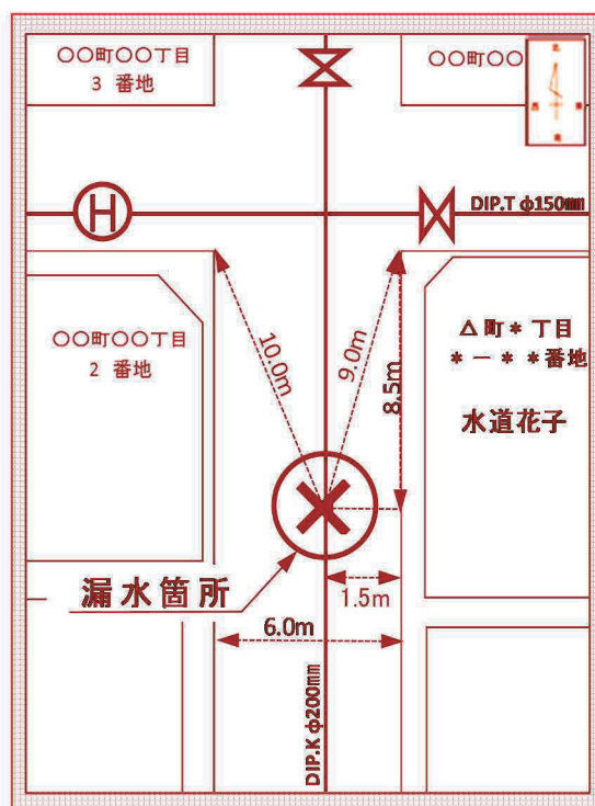
配管図 (施工後)
