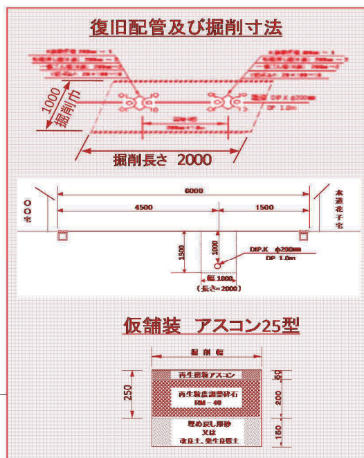
配管図 (施工後)
